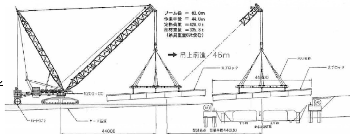
前進架設概略図
