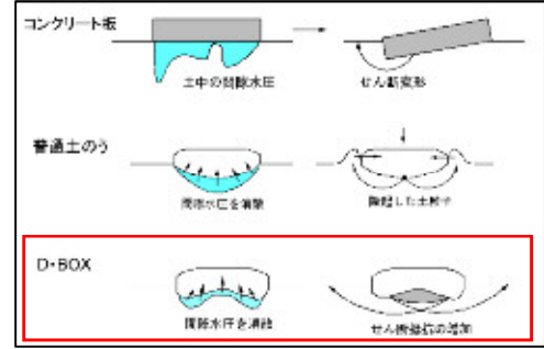
「内部拘束機能を持つ袋詰め工法」の基本的な原理
