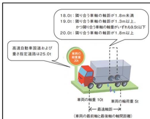
総重量と軸重の一般的制限値 (イラスト出典:特殊車両通行ハンドブック 2025.5)
