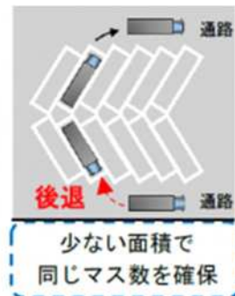
【E1A 新東名 清水 PA 下りの駐車マス拡充前後のレイアウト図】
