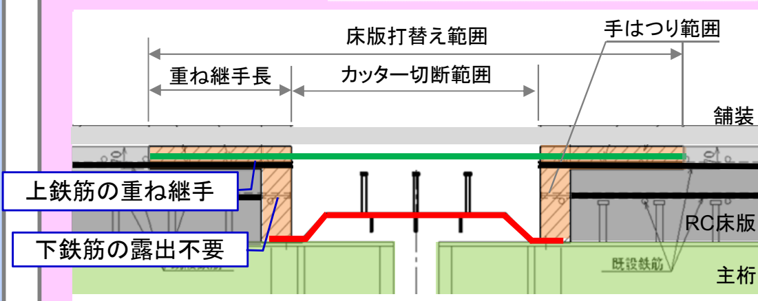
連結部橋軸断面図
