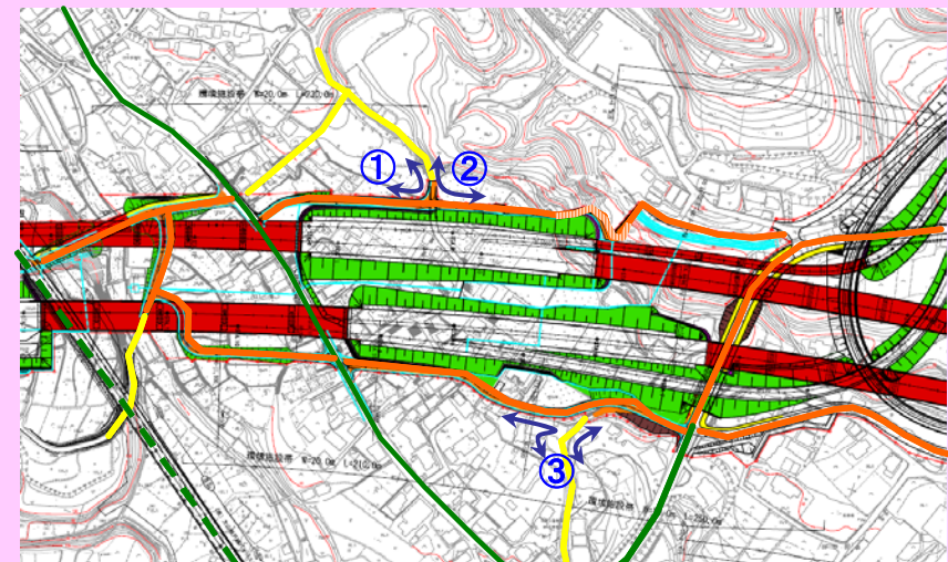
橋梁から土工への構造変更計画
