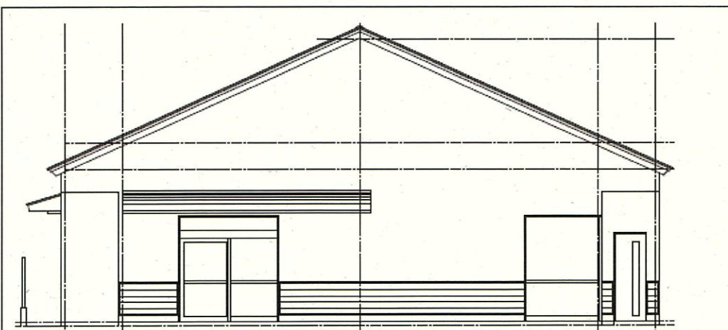
東側立面図
