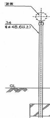
①視線誘導標 155本
