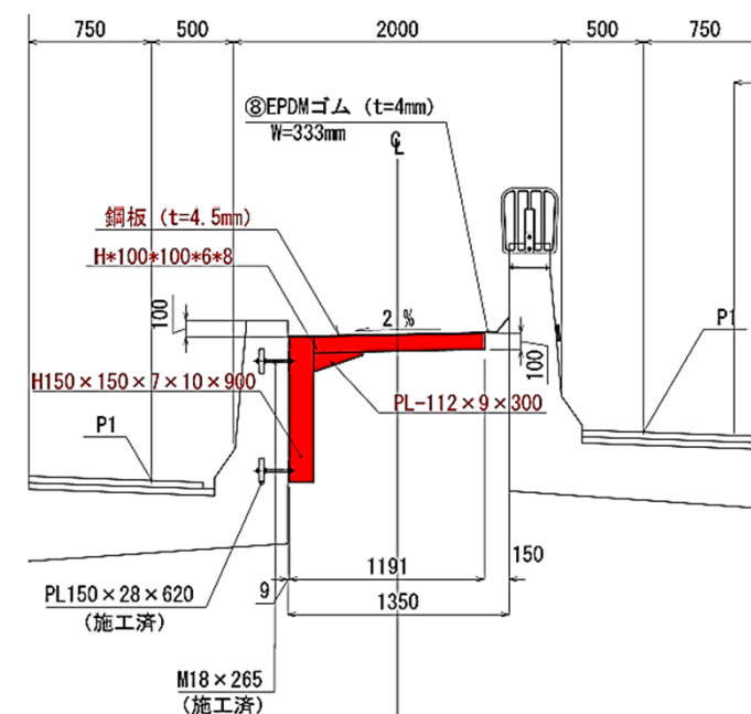
閉塞板の構造図
