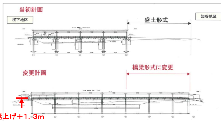
仮栈橋の構造変更
